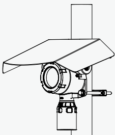
Sunshade/Deluge protection
